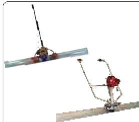
RVB1-H COD: BT1004944 Riglă vibrantă cu un mâner Motor Honda GX35, 7.000 rpm *Nu include rigla
